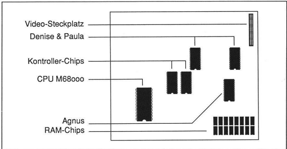
Bild 11.2: Die rechte Seite der Hauptplatine
