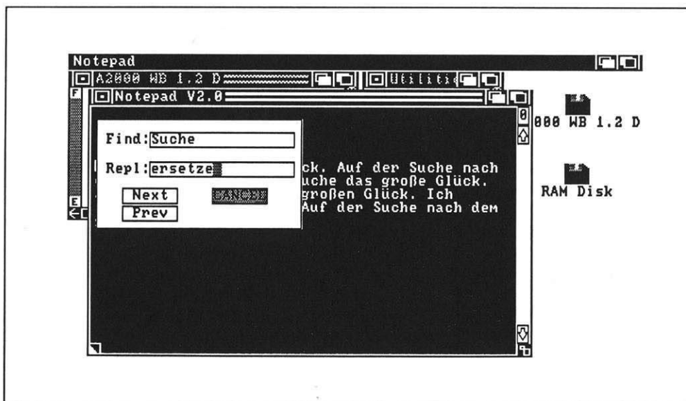
Bild 4.10: Der Find-Requester
