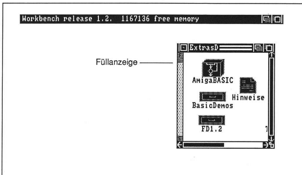
Bild 3.13: Die Disketten-Füllanzeige
