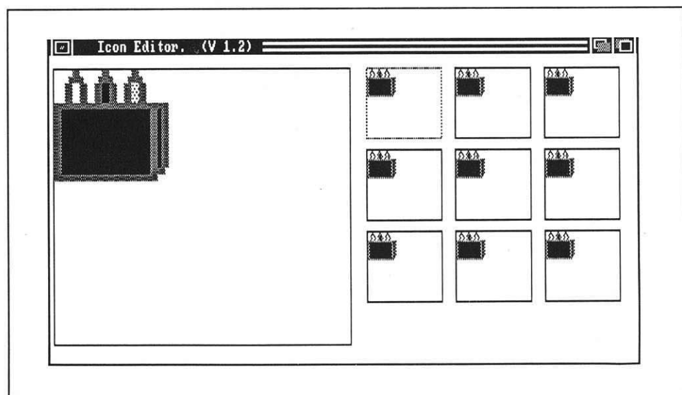
Bild 5.13: Der Piktogramm-Editor
