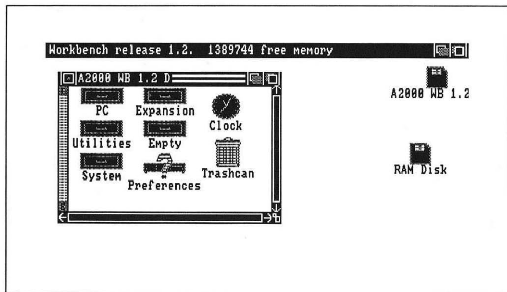
Bild 2.7: Ein Fenster
