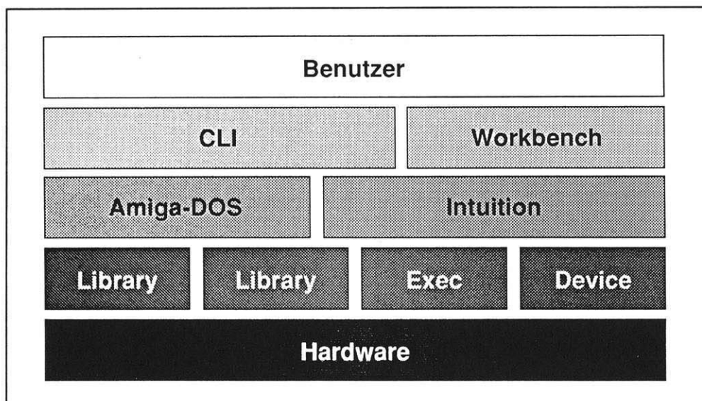
Bild 17.1: Grundriß der Amiga-Systemsoftware
