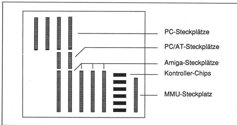
Bild 11.3: Die linke Hälfte der Hauptplatine
