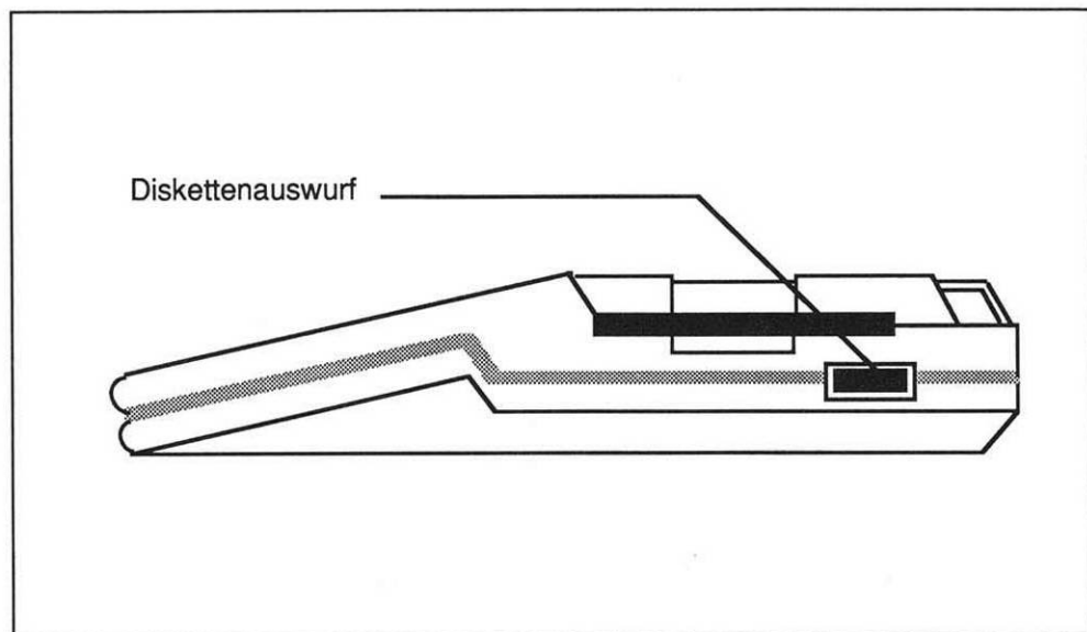
Bild 2.2: Ein Amiga-Diskettenlaufwerk
