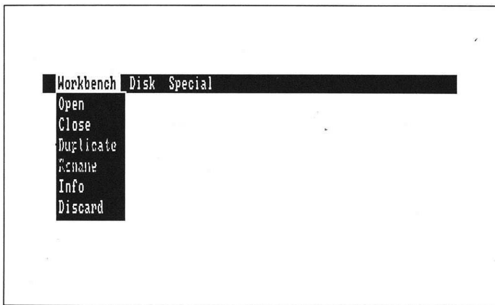
Bild 2.6: Das Workbench-Menü
