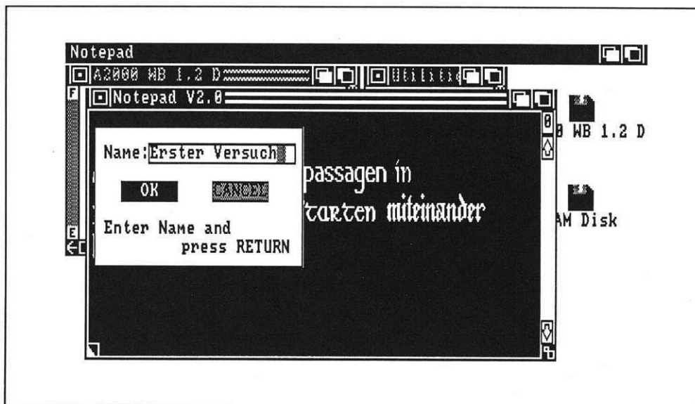
Bild 4.15: Der Save-Requester
