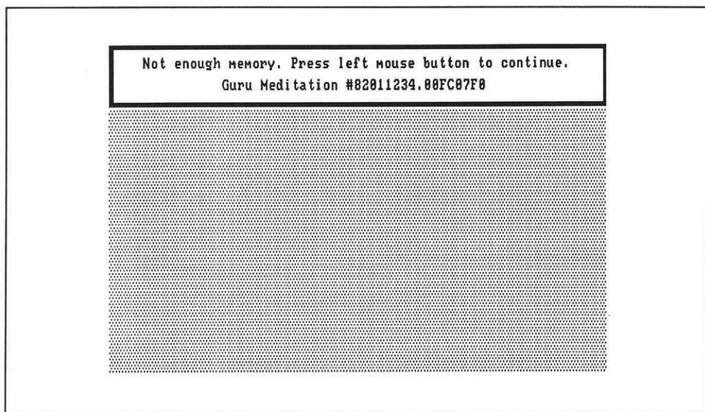
Bild 3.4: Ein Alert
