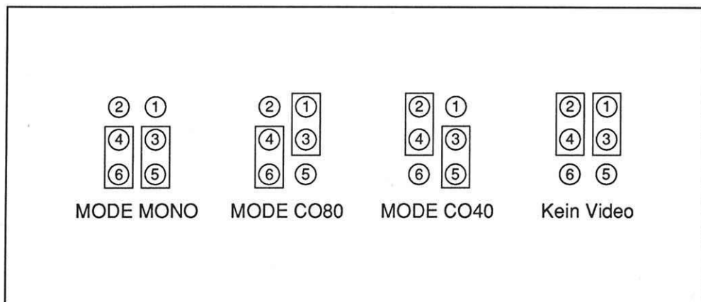
Bild 12.3: Mögliche Einstellungen des Jumperblocks J1 auf der PC-Karte
