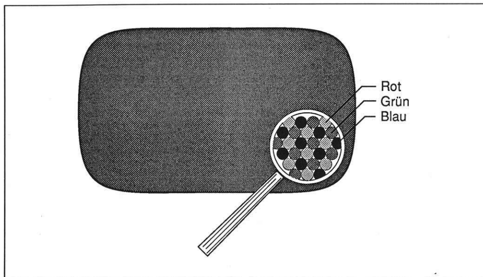
Bild 14.3: Das Grundprinzip des Farbmonitors (und des Farbfernsehers)
